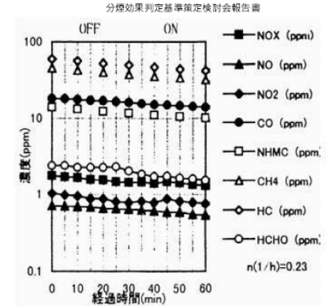
図3 実験的に発生させたガス状物質に対する空気清浄機の効果
