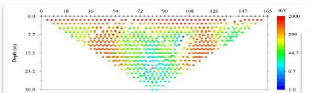
綜合電阻值分布
