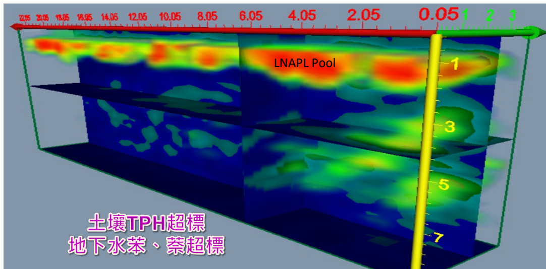
南部某工廠雜酚油分布 (3D-GPR)
