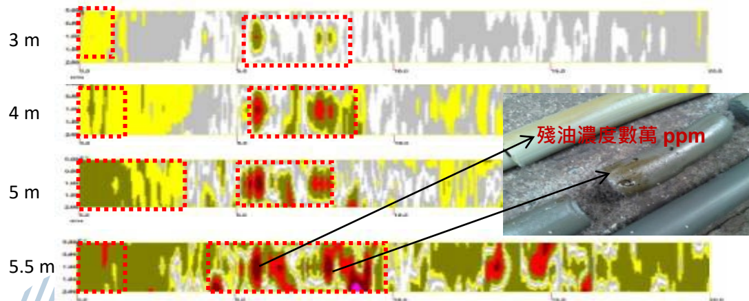
南部某工廠雜酚油分布 (3D-GPR)
